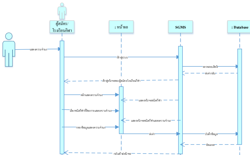
ภาพที่ 3-10 แผนภาพแสดง Sequence Diagram เพิ่มข้อมูล
