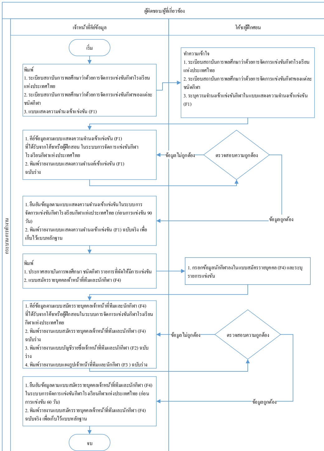
ภาพที่ 3-4 แผนภาพแสดงขั้นตอนการทำงานในส่วนการสมัครเข้าแข่งขัน
