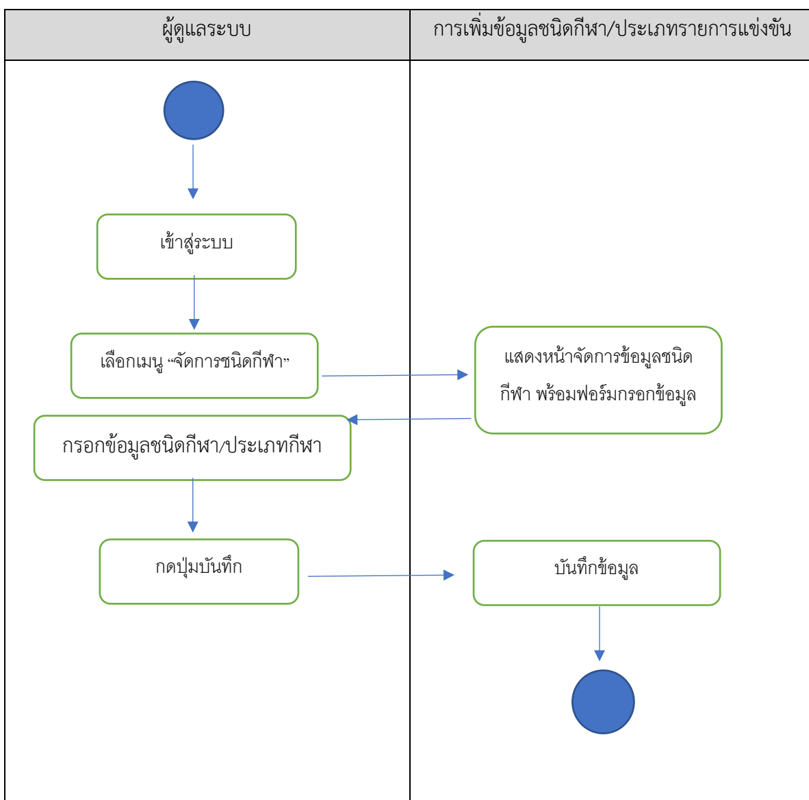
ภาพที่ 3-2 ขั้นตอนการเพิ่มข้อมูลชนิดกีฬาและประเภทรายการแข่งขัน
