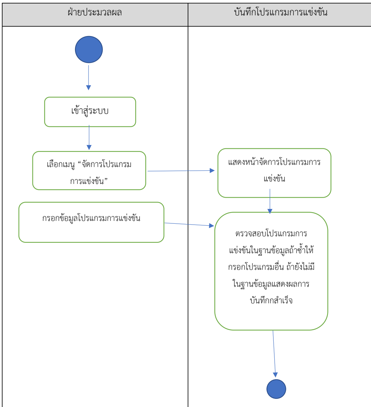
ภาพที่ 3-7 ขั้นตอนการสร้างโปรแกรมการแข่งขัน
