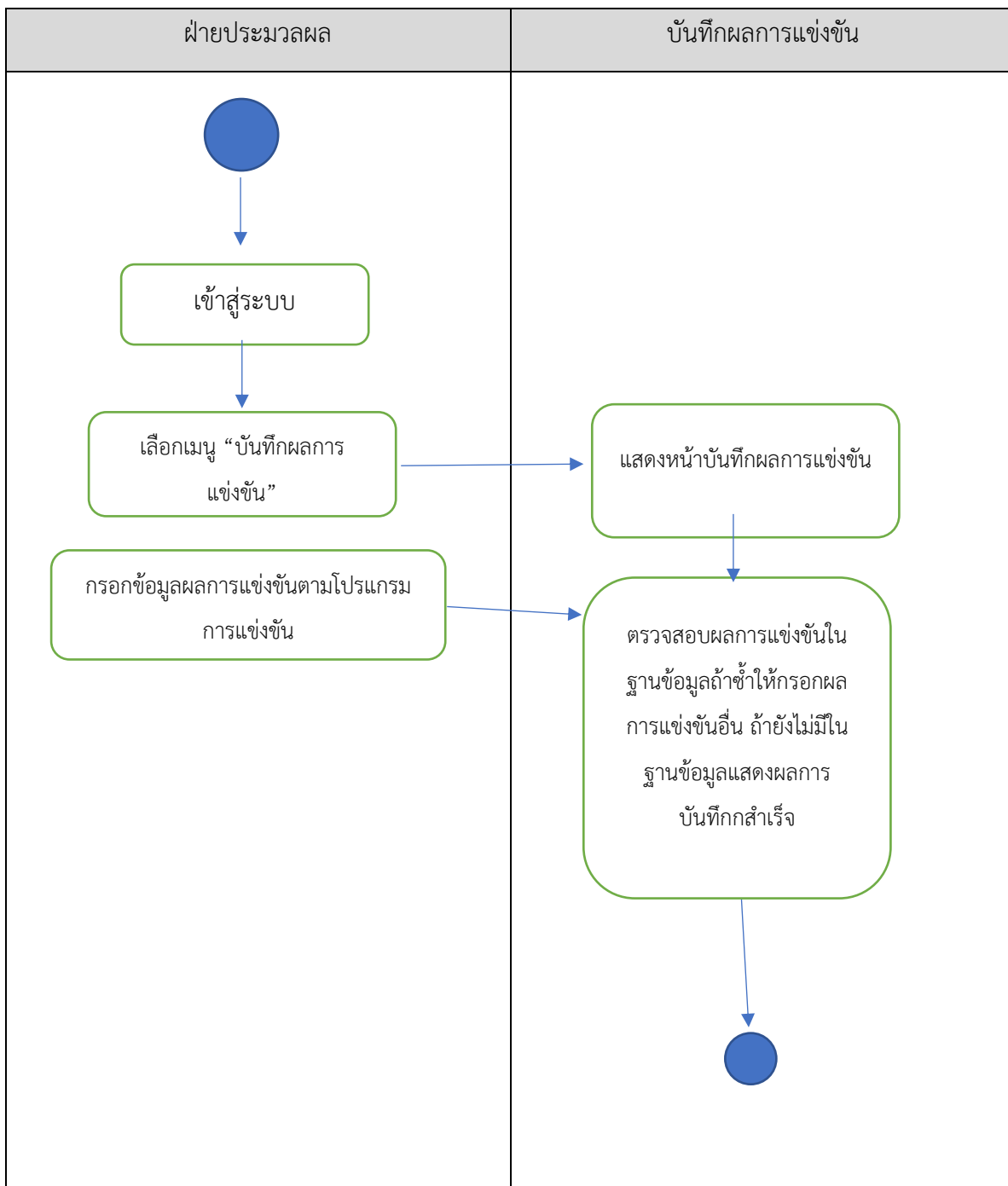
ภาพที่ 3-8 ขั้นตอนการบันทึกการแข่งขัน
