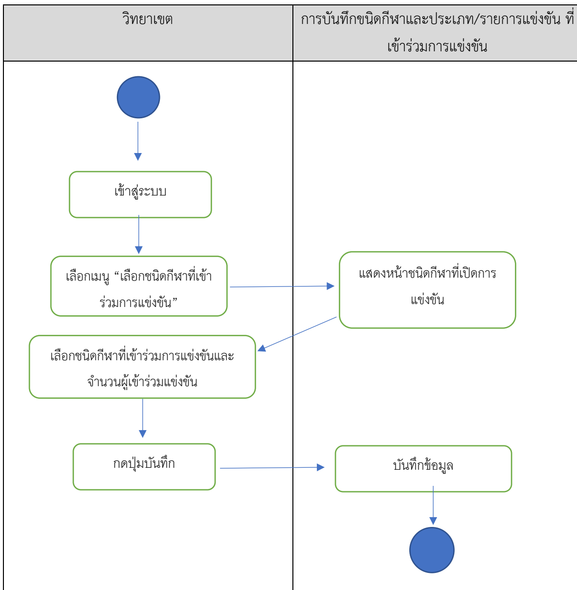
ภาพที่ 3-3 ขั้นตอนการบันทึกชนิดกีฬาและประเภท/รายการแข่งขัน ที่เข้าร่วมการแข่งขัน
