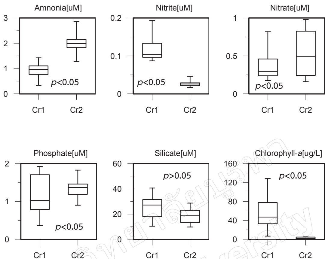
ภาพที่ 3 Box and Whisker plots ของข้อมูลแอมโมเนีย ไนไตรท์ ไนเตรท ซิลิเกต ฟอสเฟต ซิลิเกต และคลอโรฟิลล์-เอ ในช่วงของการเก็บตัวอย่างเดือนมีนาคม (Cr1) และเดือนสิงหาคม (Cr2) พ.ศ. 2552
