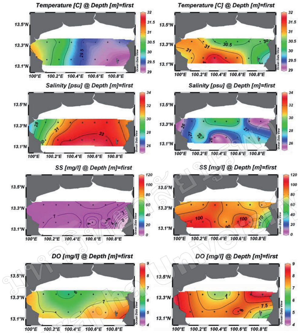
ภาพที่ 4 การแพร่กระจายที่ผิวทะเลของอุณหภูมิ ความเค็ม สารแขวนลอยทั้งหมดในน้ำ และออกซิเจนละลายน้ำในช่วงของการเก็บตัวอย่างในเดือนมีนาคม และ สิงหาคม พ.ศ. 2552 จุดแสดงสถานีตรวจวัดคุณภาพน้ำ
