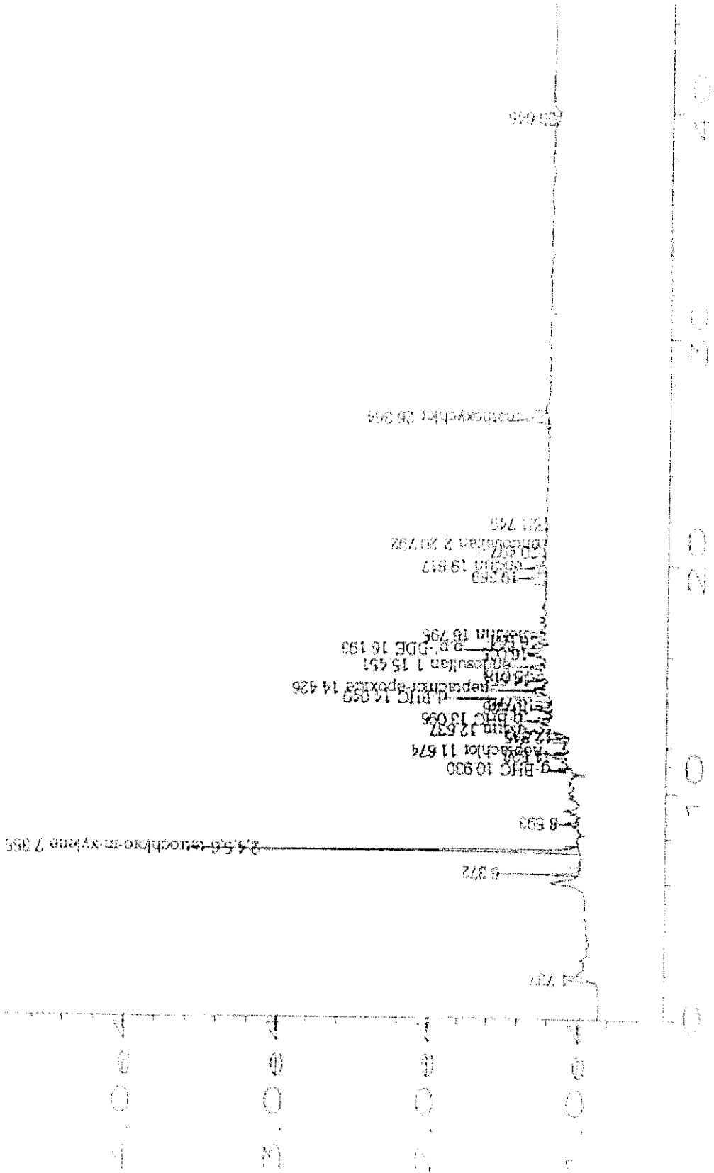
ภาพที่ 54 โครมาโตแกรมของสารปราบศัตรูพืชและสัตว์กลุ่มออร์กาโนคลอรัในหอยนางรม
