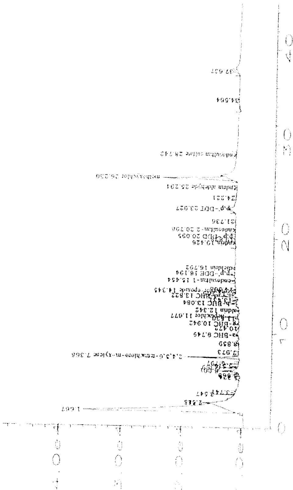
ภาพที่ 56 โครมาโตแกรมของสารปราบศัตรูพืชและตัวกลุ่มออกกราโนคลอรีนในแหล่งกักตุน
