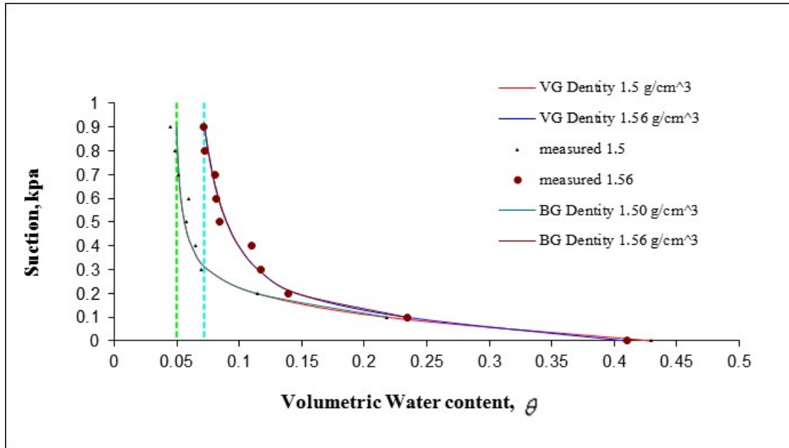
รูปที่ 3-27 กราฟแสดงความสัมพันธ์ระหว่าง volumetric water content กับ ค่าแรงดูด (Suction) ของ แก๊สไซฮอลล์ E20 กับอากาศ ที่ความหนาแน่น 1.50 g/cm 3 และความหนาแน่น 1.56 g/cm 3
