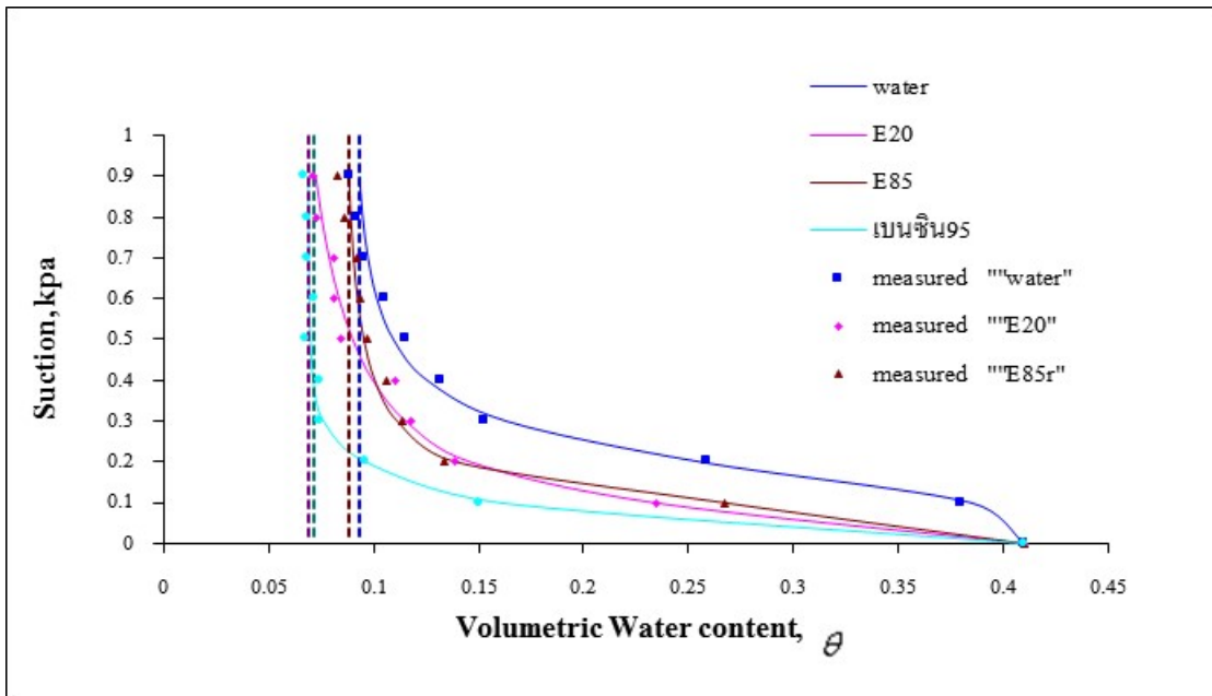
รูปที่ 3-35 กราฟแสดงความสัมพันธ์ระหว่าง Volumetric water content กับ ค่า Suction ของน้ำกลั่น มันเบนซิน 95 แก๊สโซฮอล์ E20 และ แก๊สโซฮอล์ E85 กับอากาศที่มีความหนาแน่น 1.56 g/cm 3 (VG Model)
