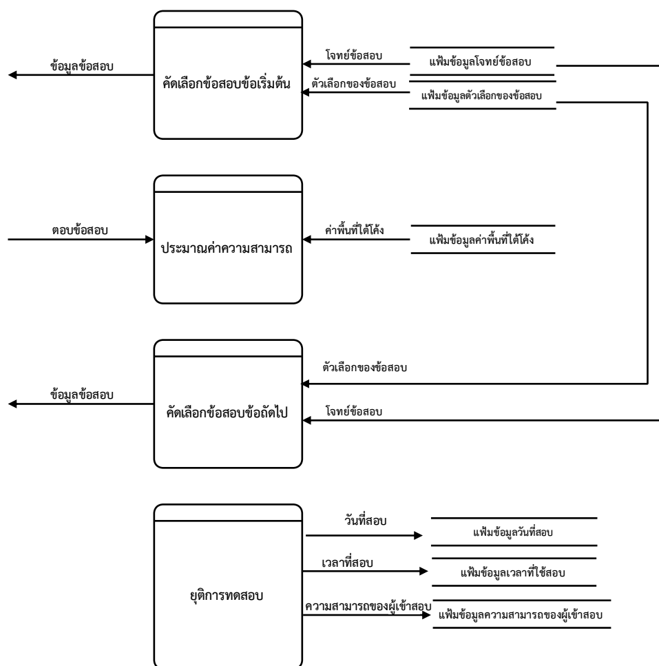
ภาพที่ 33 แผนผังการไหลของข้อมูลระดับ 1 (Data Flow Diagram Level 1) ของกระบวนการจัดการทดสอบ
