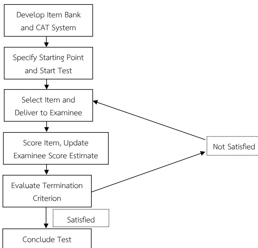
ภาพที่ 10 ขั้นตอนการดำเนินการทดสอบแบบปรับเหมาะด้วยคอมพิวเตอร์ (Thompson & Weiss, 2011, p. 2)
