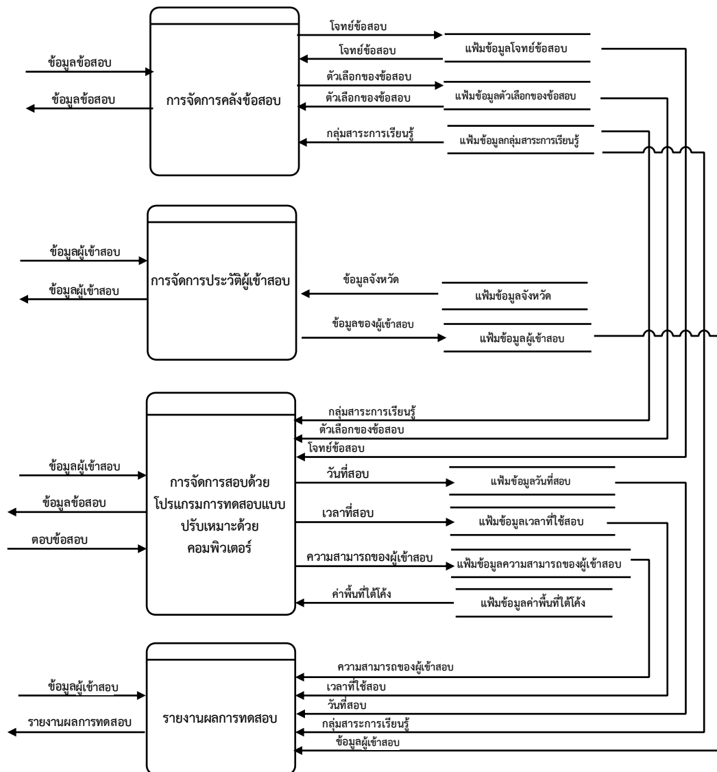
ภาพที่ 31 แผนผังการไหลของข้อมูลระดับ 0 (Data Flow Diagram Level 0: DFD 0) ของโปรแกรมการทดสอบแบบปรับเหมาะด้วยคอมพิวเตอร์
