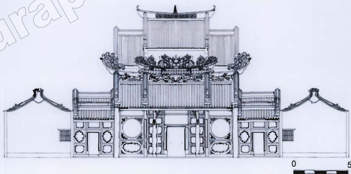
ภาพภาคผนวก ค-4 ภาพลายเส้นรูปด้านหน้า (วิหารหน้า) วัดจีนประชาสโมสร (วัดเล่งฮกยี่)
