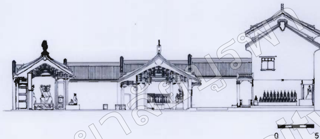
ภาพภาคผนวก ค-5 ภาพถ่ายเส้นรูปตัดด้านข้างของวิหารหน้า วิหารหลัก วิหารบูรพาจารย์ วัดจีนประชาสโมสร (วัดเล่งฮกยี่)
