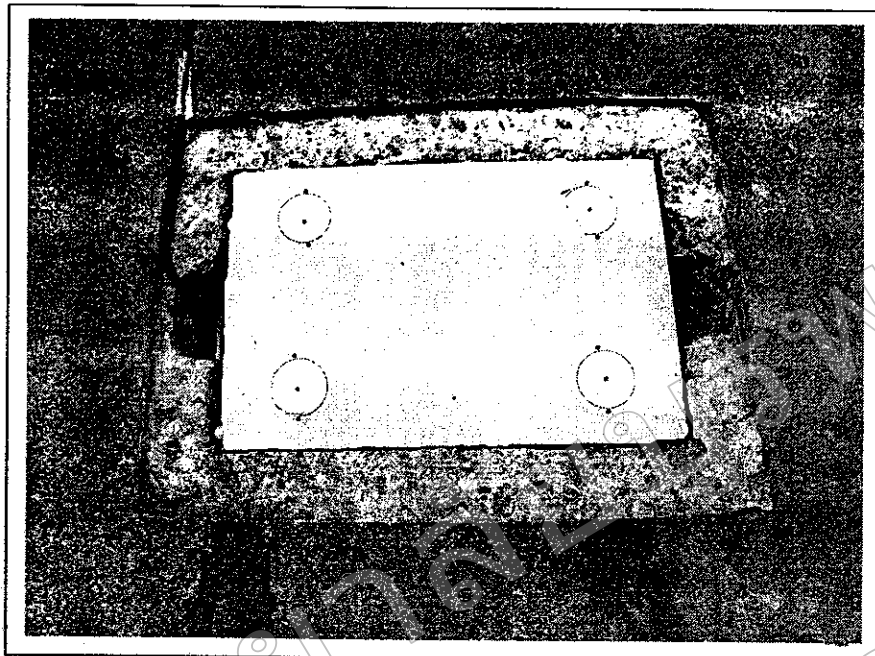
ภาพที่ 55 แผ่นวัดแรงปฏิกิริยาสามทิศทาง (Force platform)
