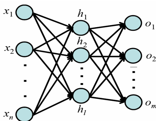
ภาพที่ 2-18 ตัวอย่างข่ายงานประสาทเทียมแบบหลายชั้น
