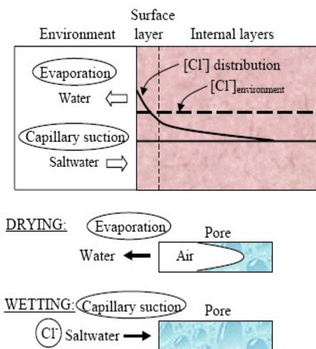
ภาพที่ 2.2 การจำลองข้อมูลการเคลื่อนที่ของคลอไรด์ในคอนกรีต ภายใต้อิทธิพลของวงจรสภาวะเปียกสลับแห้ง
