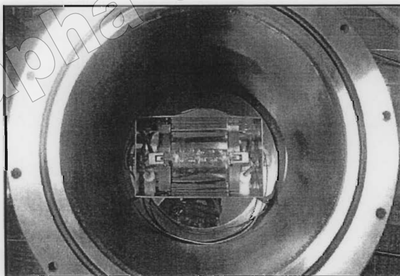
ภาพที่ 6 แสดงอุปกรณ์ให้ความร้อนด้วยหลอดฮาโลเจนภายใน Chamber ของชุดอุปกรณ์ให้ความร้อนในสุญญากาศ
