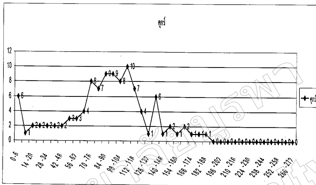
ภาพภาคผนวก ก-5 กราฟแสดงความถี่ปริมาณการใช้ตู้คอนเทนเนอร์ตาม อัตราภาคชั้นของวันศุกร์
