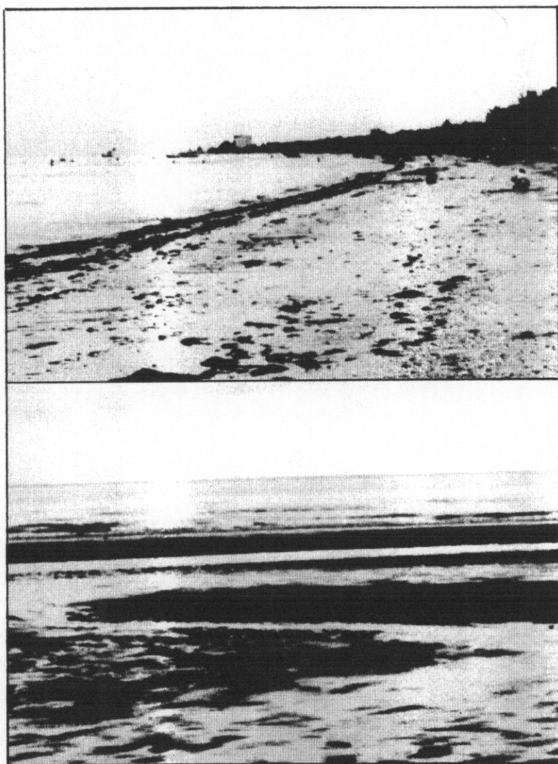
ภาพที่ 27 แสดงปัญหาที่เกิดจากยูโทรฟิเคชัน โดยพบสาหร่ายตายบริเวณชายหาด บางแสน-วอนนภา เมื่อวันที่ 23 กุมภาพันธ์ 2544
