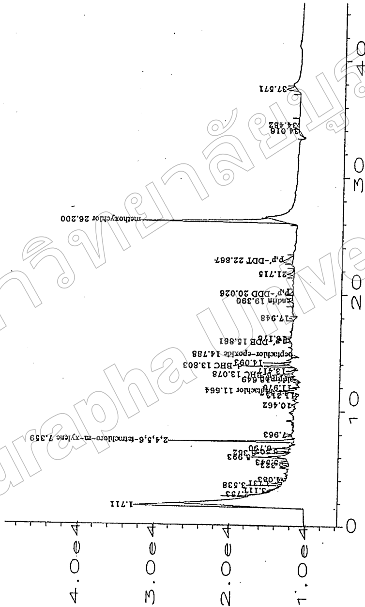
ภาพที่ 49 โครมาโทแกรมของสารกำจัดศัตรูพืชและสัตว์กลุ่มออร์กาโนคลอรีนในแมลงก้นดง
